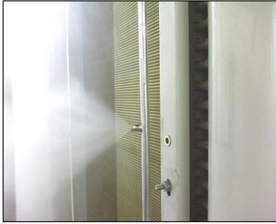
Şekil 8. Sisleme Sistemli Islak-Kuru Soğutucu [11]
