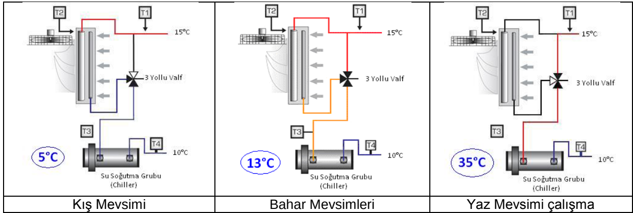
Şekil 2.A,B,C Soğutma grubu ile doğal soğutma bataryalı uygulama şematik gösterim [5]
