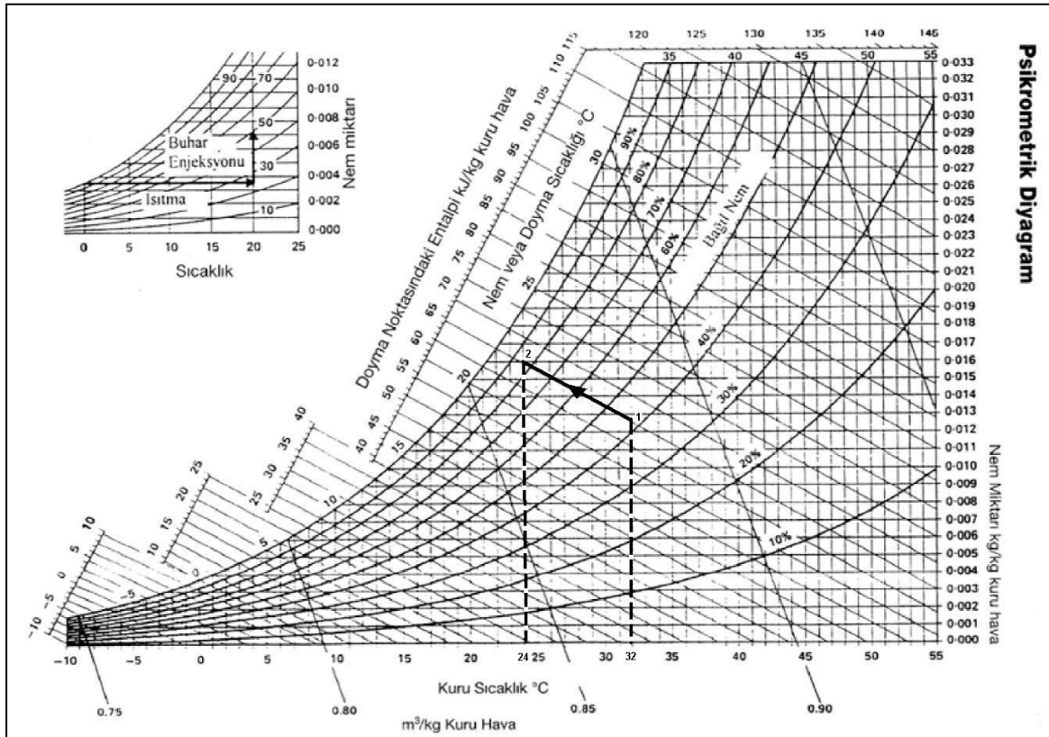
Grafik 2. Psikrometrik diyagram üzerinden örnek noktaların gösterimi [14]
