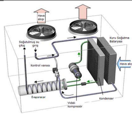
Şekil 3.B Entegre Doğal Soğutma bataryalı hava soğutmalı su soğutma grubu şematik [1]
