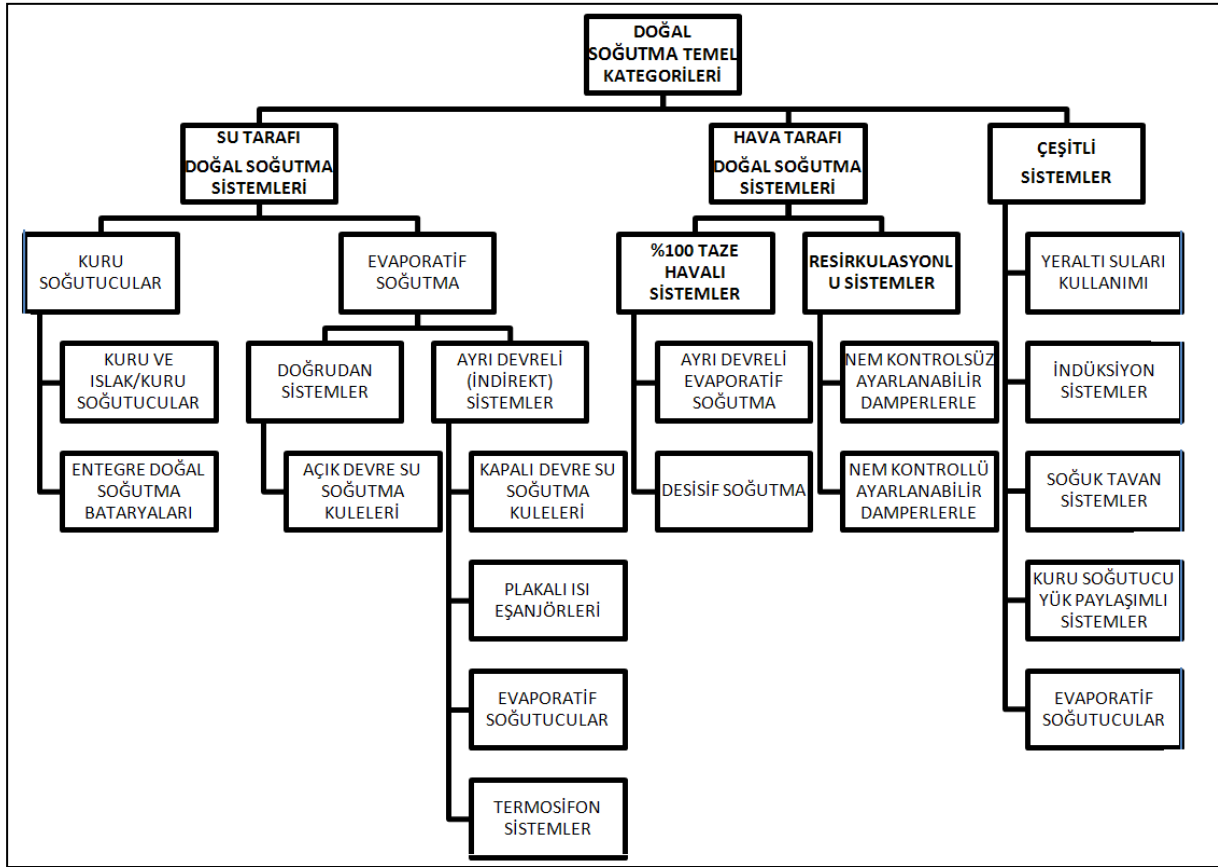
Sekil 1. Doğal Soğutma Temel Kategorileri [1]
