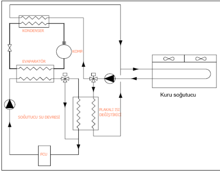
Şekil 6. Moskova'da bulunan alışveriş merkezinde kurulu kuru soğutucu prensip şeması [13]
