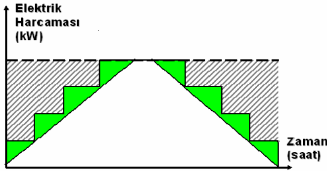
Grafik 4. Fanların step kontrol uygulanarak ihtiyaca göre devreye alındığı bir kuru soğutucuda bir günlük periyotta fanların elektrik harcaması. (Taralı alan, tüm fanların sürekli kullanılmaması sayesinde tasarruf edilen elektrik miktarını kWh olarak göstermektedir.)
